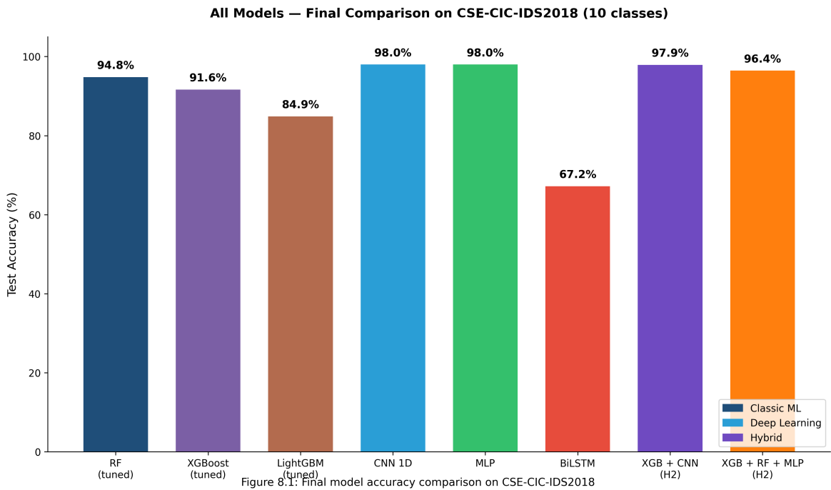
FIGURE 4.4 – Comparaison de la précision finale des modèles sur CSE-CIC-IDS2018
